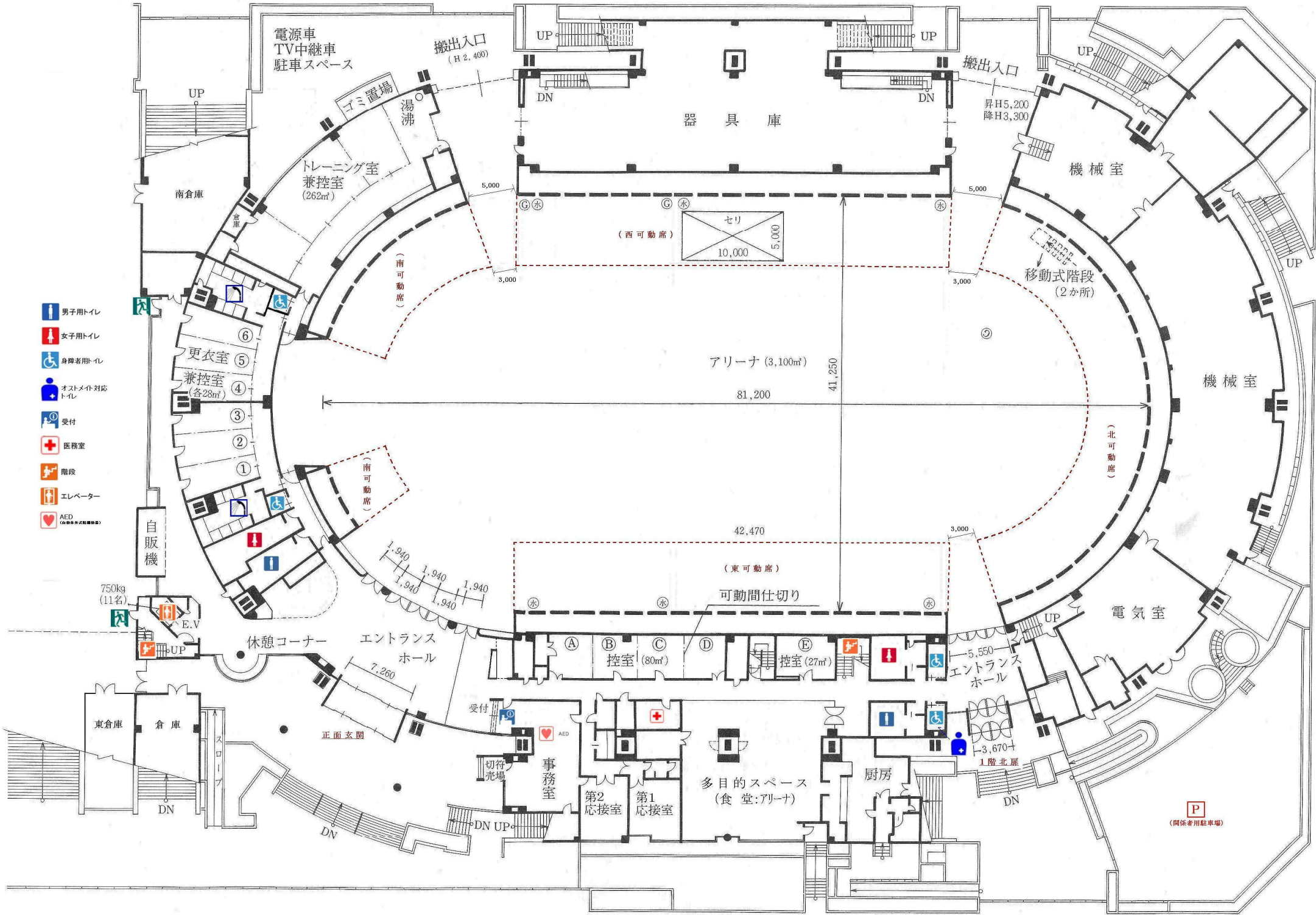
1階平面図
